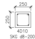
DETAIL K1A SKALA 1:20
