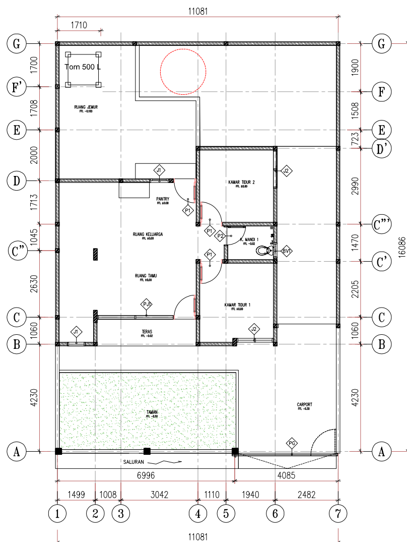
RUMAH JALAN KARYAWAN I No.6 Denah Posisi Kusen Pintu & Jendela Skala 1:100 Utara
