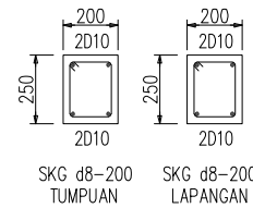
POTONGAN TB1 SKALA 1:20
