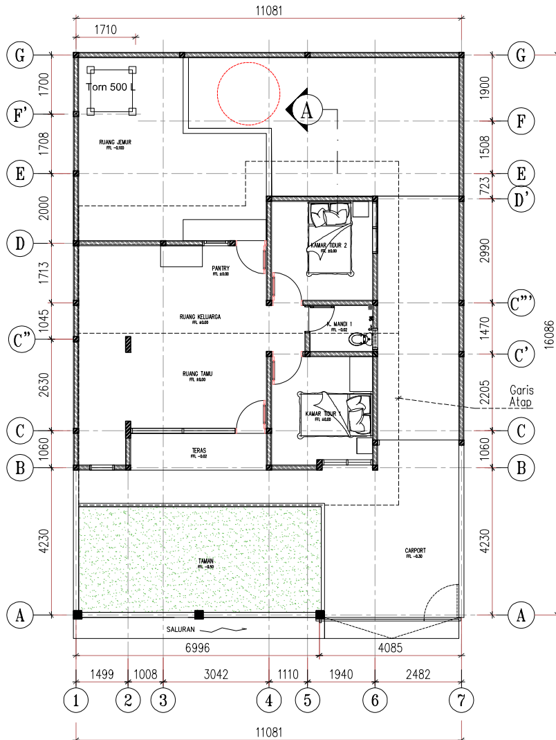
RUMAH JALAN KARYAWAN I No.6 Denah Rencana Lantai Dasar Skala 1:100
