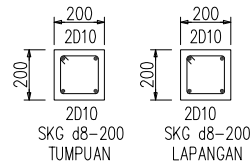
POTONGAN RB2 SKALA 1:20
