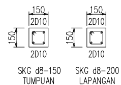
POTONGAN RB2 SKALA 1:20
