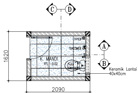
Denah K. Mandi 1 Skala 1:50
