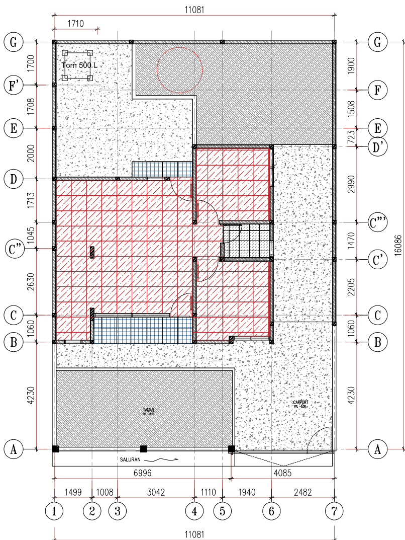
RUMAH JALAN KARYAWAN I No.6 Denah Finishing Lantai Skala 1:100
