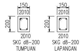
POTONGAN RB1 SKALA 1:20
