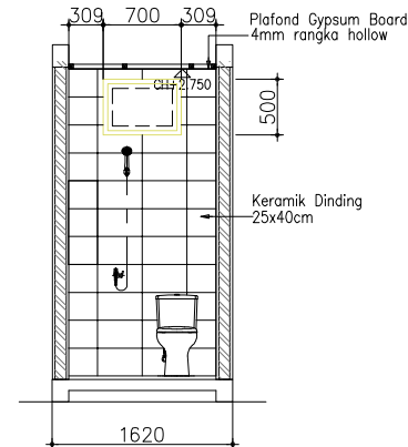
Potongan D Skala 1:50
