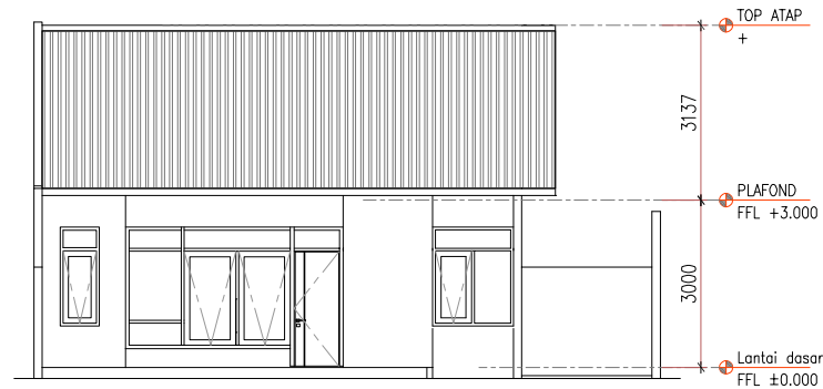
RUMAH JALAN KARYAWAN I No.6 Tampak Depan Skala 1:100
