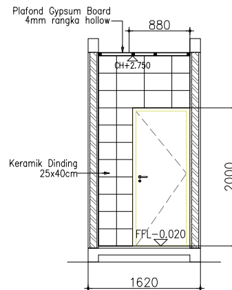
Potongan C Skala 1:50
