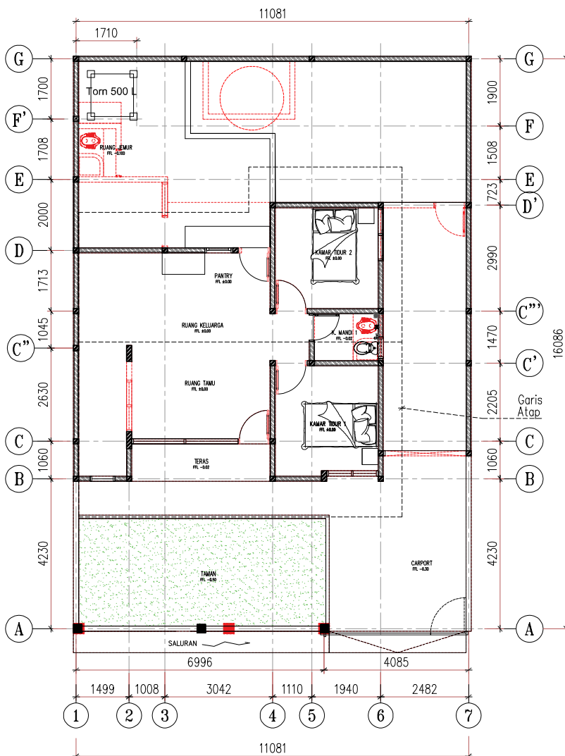
RUMAH JALAN KARYAWAN I No.6 Denah Superimposed & Pembongkaran Skala 1:100 Utara
