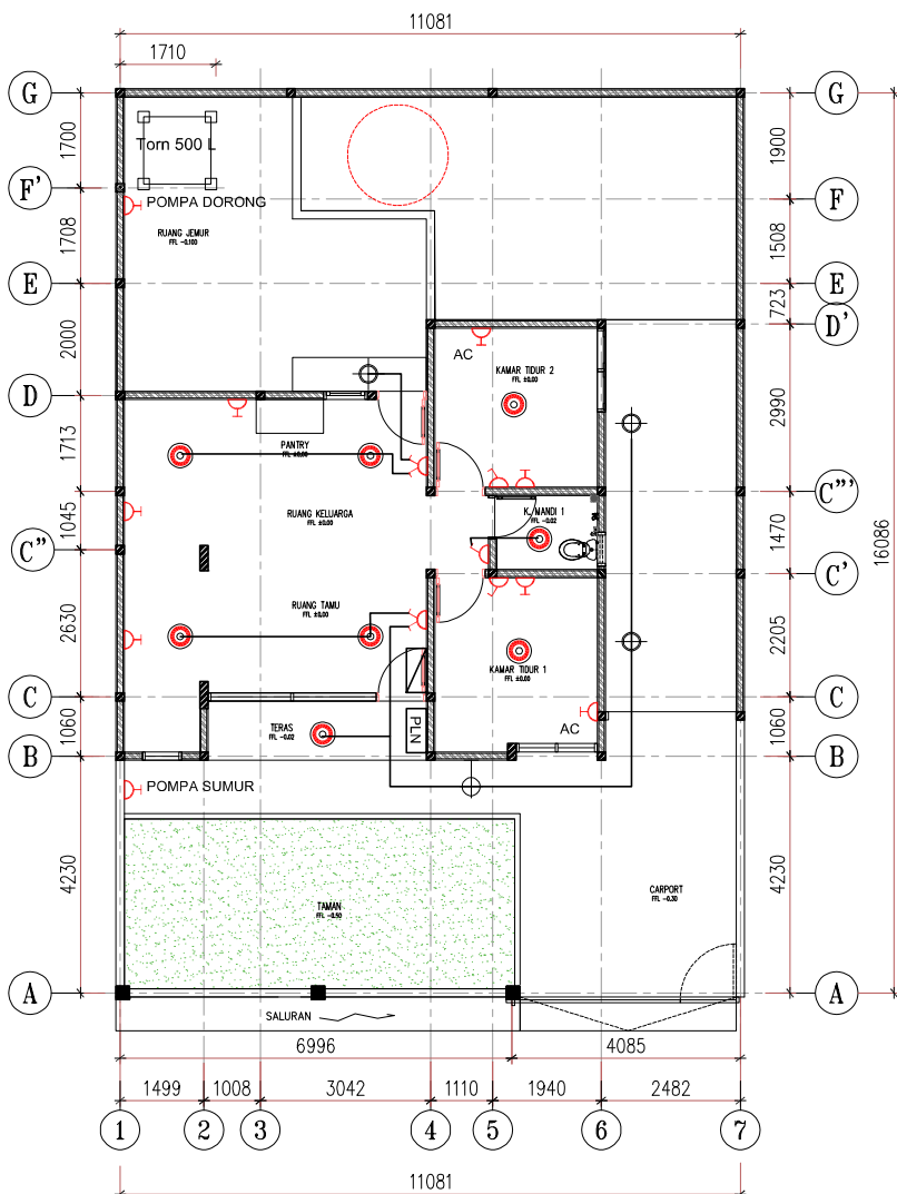
RUMAH JALAN KARYAWAN I No.6 Denah Penerangan & Power Skala 1:100
