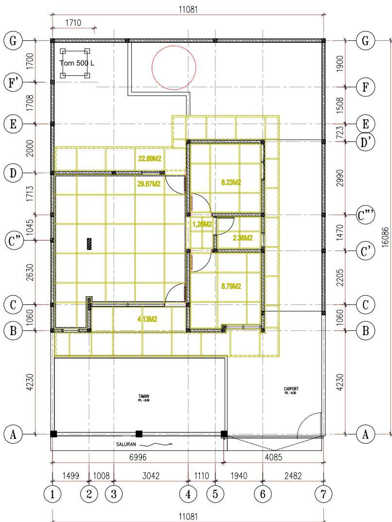
RUMAH JALAN KARYAWAN I No.6 Denah Rangka Plafond Skala 1:100
