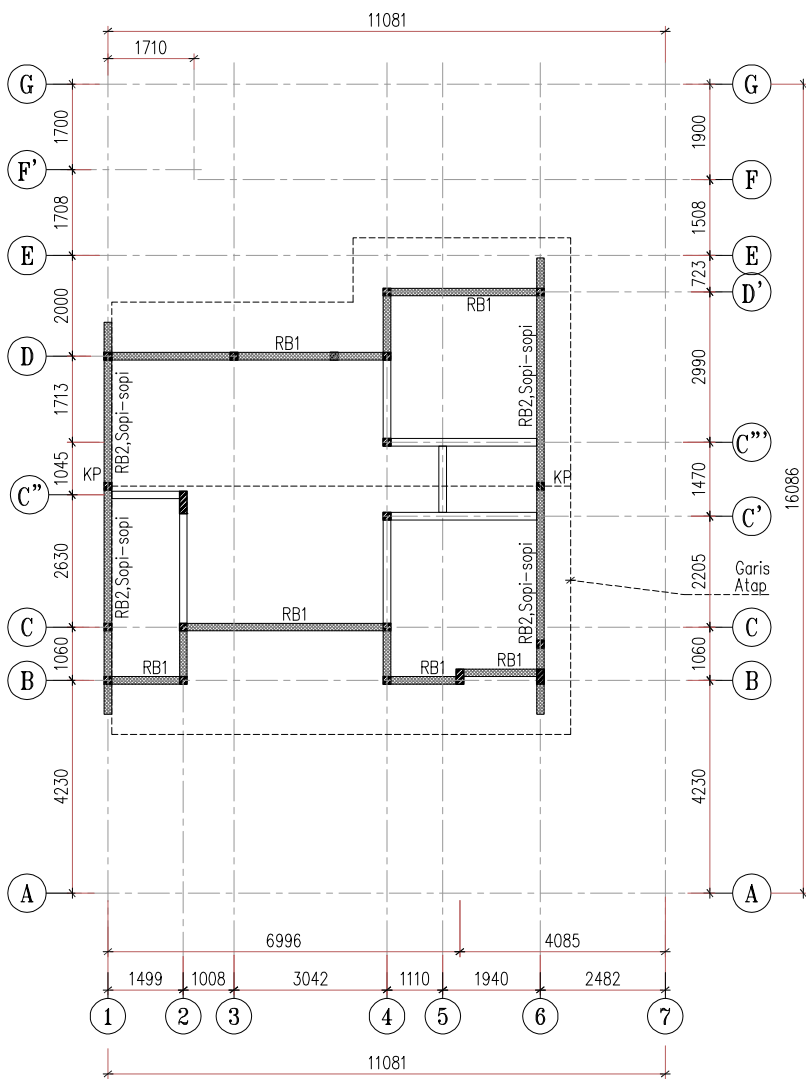
RUMAH JALAN KARYAWAN I No.6 Denah Rencana Struktur Skala 1:100
