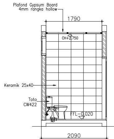
Potongan B Skala 1:50
