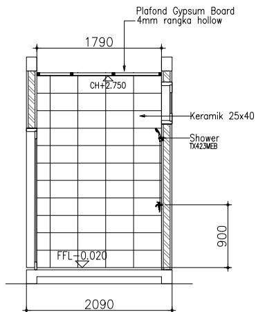
Potongan A Skala 1:50
